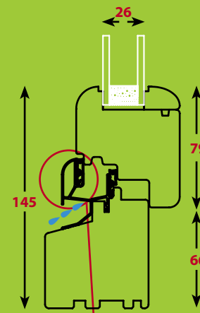
NODO INFERIORE NOED INFÉRIEUR
