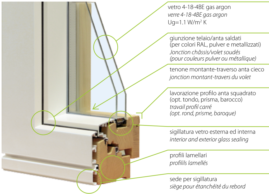
NODO CENTRALE NOED CENTRAL
