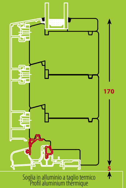
NODO INFERIORE PORTAFINESTRA NOED INFÉRIEUR PORTE - FENÊTRE
